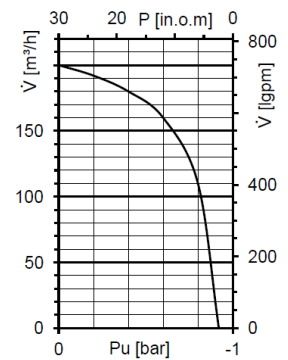
Charakterystyka pomp próżniowej
