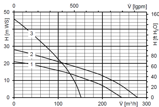
Charakterystyka pomp wodnych
